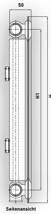
Seitenansicht
