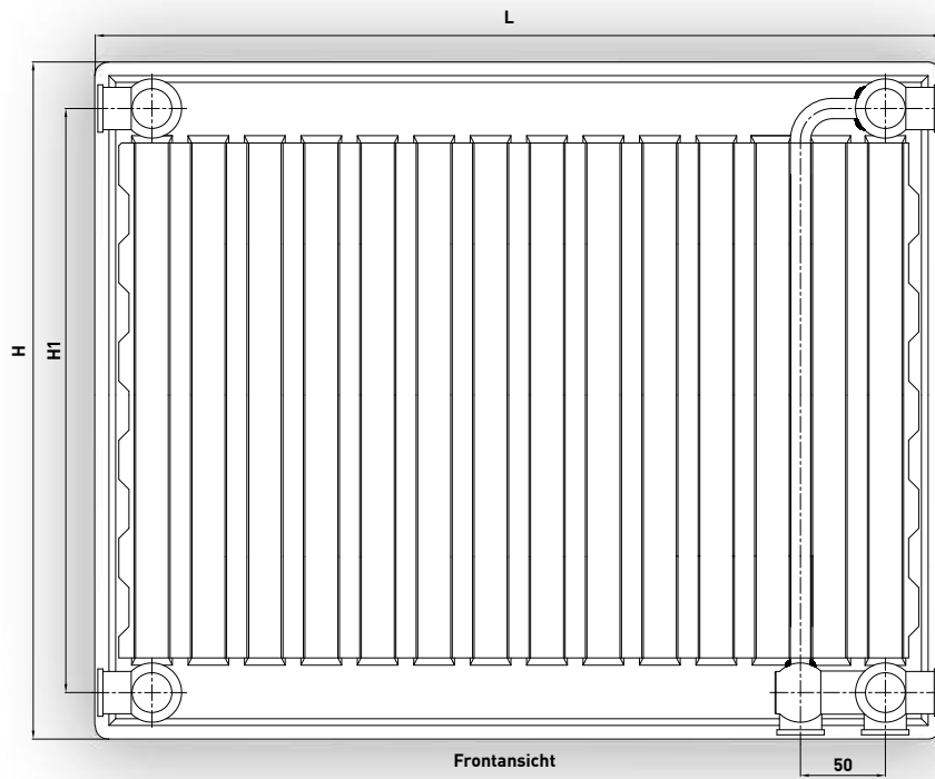
Frontansicht
