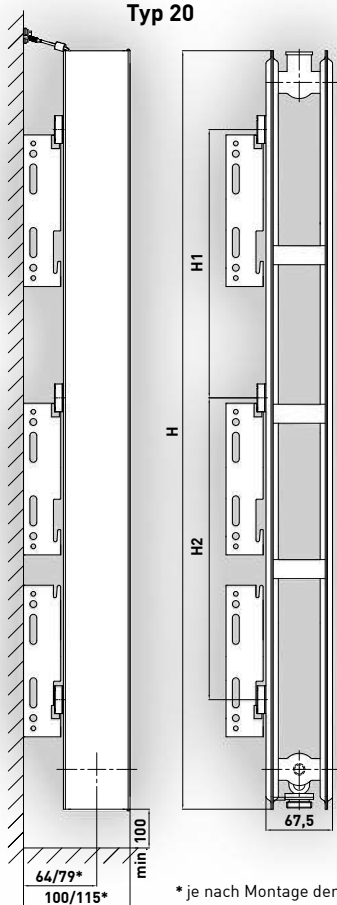
Typ 20
